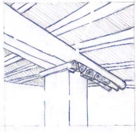
التسقيف بالقصب
