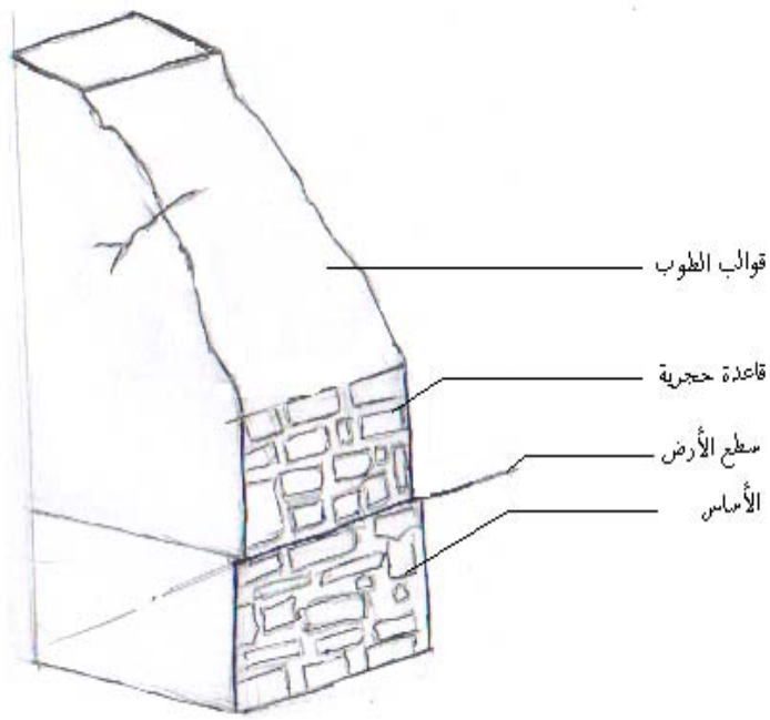
رسم تخيلي يوضح طريقة وضع الحجارة و قوالب الطوب
