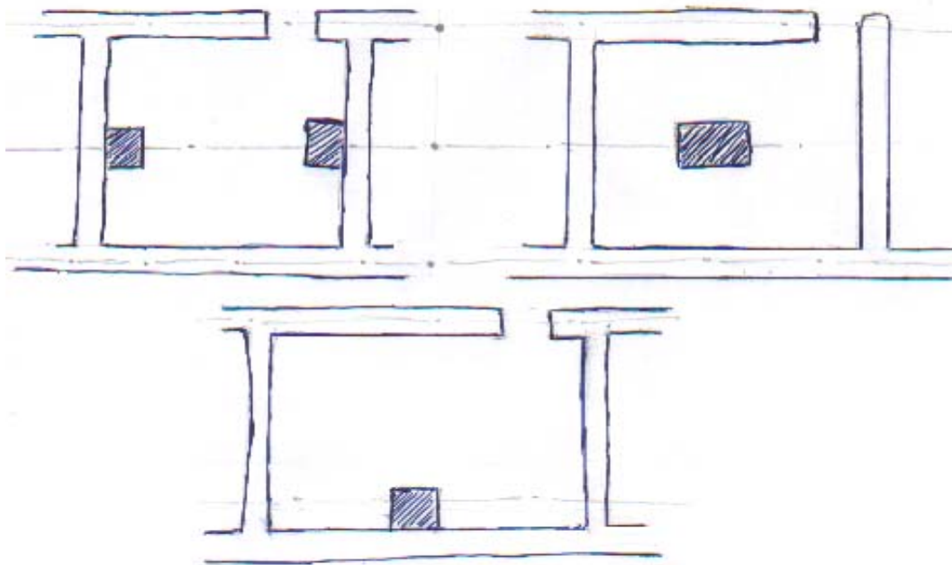
الشكل رقم ( 9 ) رسم تخطيطي يوضح كيفية وضع الدعامات وتوزيعها ( عن الطالب )
